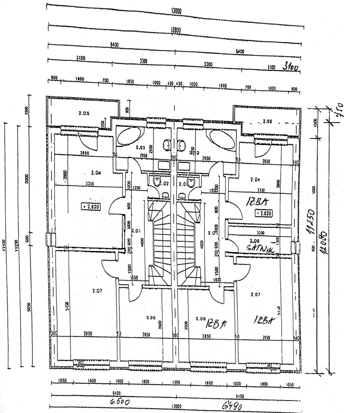
Rôdorys 2 NP
